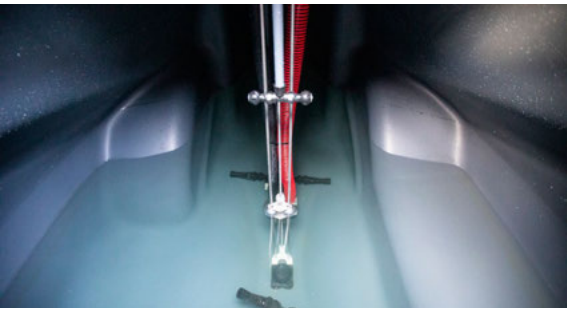
Leeb 4 AX Tankinnenansicht: kraftvolle Rühr- und Reinigungsdüsen
