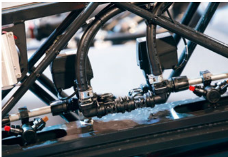
HORSCH Leeb 4 AX – elektrische Düsenschialtung
