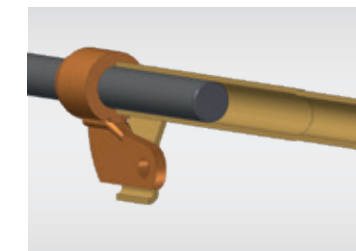
Passgenaue Verbindung durch das aufgeweitete Rohr
