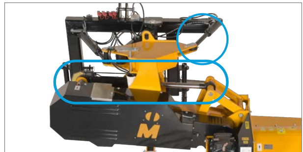
Die hydraulische Non-Stop Anfahrssicherung schwenkt das Mulchgerät im Ernstfall effektiv aus dem Kollisionsbereich.
