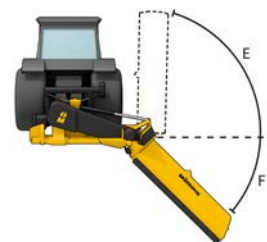
Arbeits-/Verschiebepbereiche (cm)
