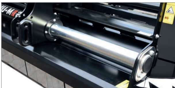
Die hydraulische Seitenverschiebung verfügt über kunststoffgelagerte Verschieberohre für ein verschleißarmes Arbeiten im Dauereinsatz.
