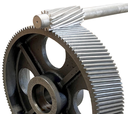
Zahnräder mit Schrägverzahnung (ab SRW 397) Roues dentées à denture hélicoïdale (à partir de SRW 397)
