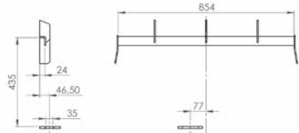
Weidmann Plattenaufnahme
