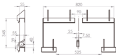
Schäffer Plattenaufnahme
