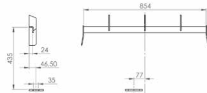
Weidemann Plattenaufnahme
