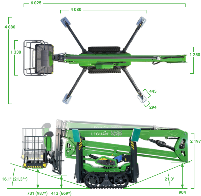
Maße in Millimetern. *Maximale Werte für erhöhte Fahrposition (EDP).
