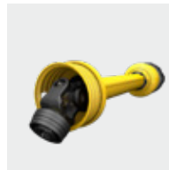
Zapfwellendrehzahl 540 / 1.000 U/min
