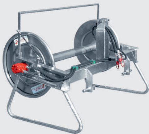
Schlauchhaspel SHW 400 mit Hydraulik-Antrieb und Dreipunktaufhängung
