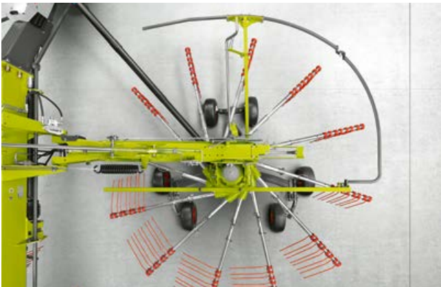
Hydraulische Vorgewendeanschlätze.
