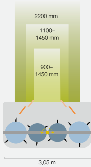
3200 CONTOUR
